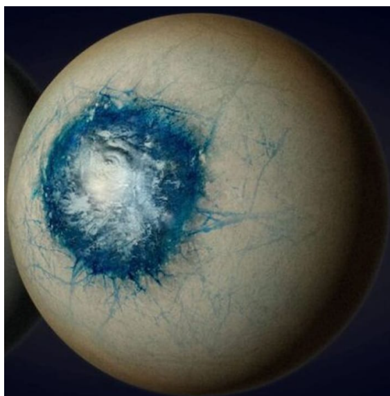
(d) LHS 1140 b ( d_M = 2.779 , 74.3th percentile)
